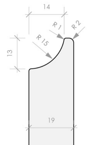
verticale snede
