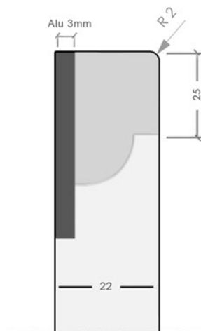
verticale snede
