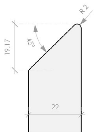
verticale snede
