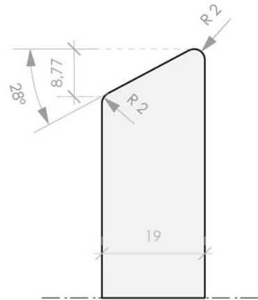
verticale snede
