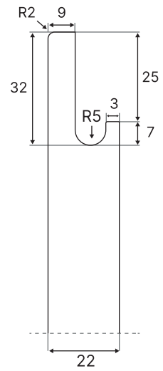
verticale snede
